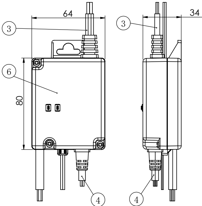
正面図
