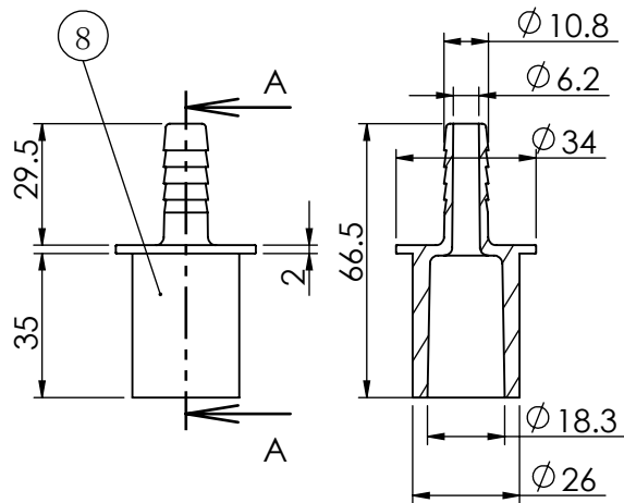
断面図 A-A
